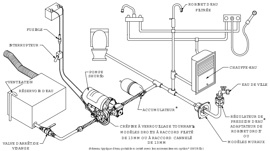
(Réseau typique d'eau potable monté avec les accessoires en option* SHURflo)
